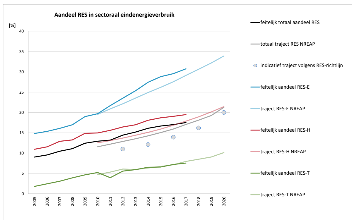
Figuur 1: Daadwerkelijke en geplande aandelen van hernieuwbare energie voor de EU-28 (2005-2020, %). Bron: Eurostat en de nationaal actieplannen voor energie uit hernieuwbare bronnen (NREAP's)
